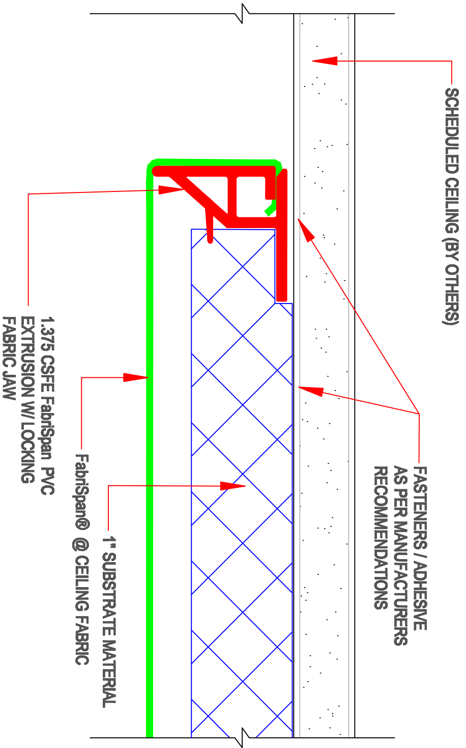
7 1.375 CSFE Edge Detail - Bottom Load Scale: 1:1 Reference: Edge Detail
